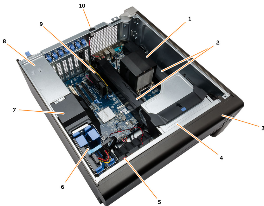
图 1: T3610 计算机内部视图
